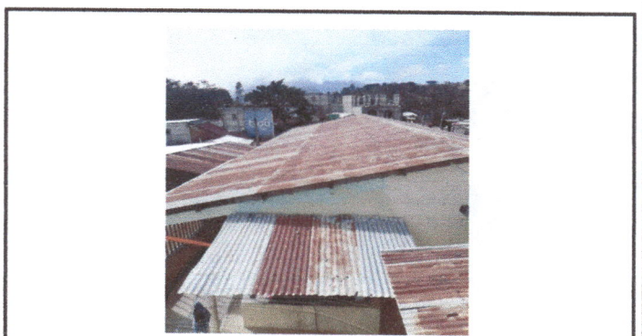
Foto 6: Sustitucion de lamina por lamina troquelada aluzinc calibre 26
